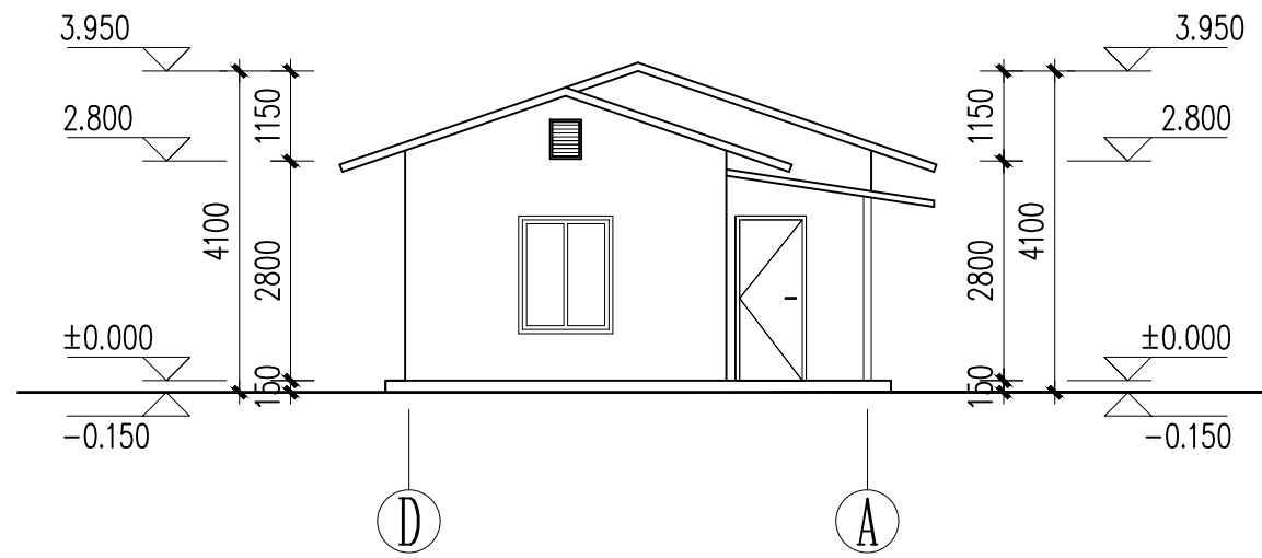
D-A Axis Elevation 1:100
