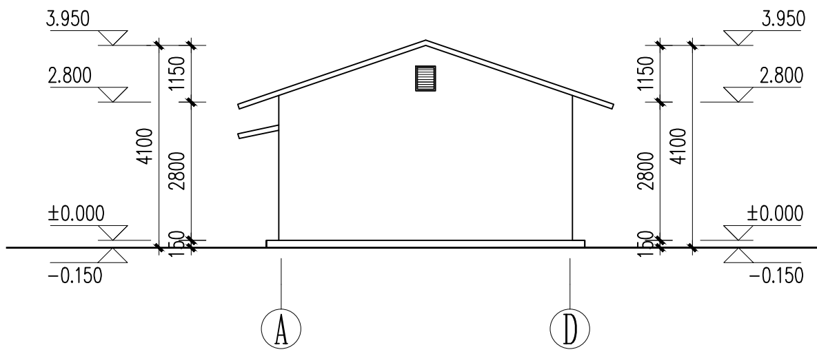
A-D Axis Elevation 1:100
